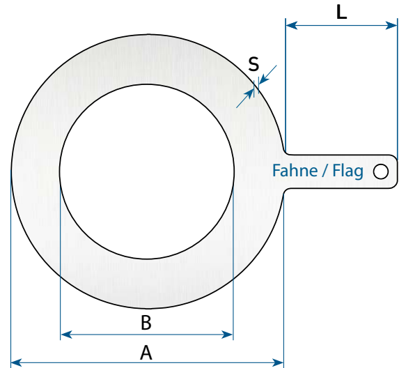
Ringscheiben Typ LS / Ring spacer Type LS
