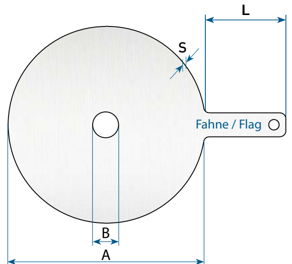
Drosselscheiben Typ DS / Orifice plate Type DS
