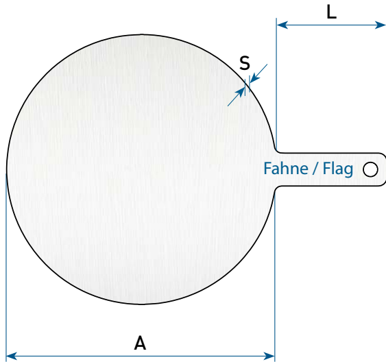
Blindscheiben Typ BS / Blank disks Type BS
